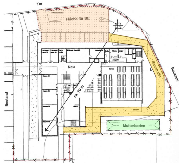
Baustelleinrichtung planen.
