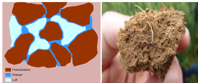
Böden sind poröse Körper aus Festsubstanz und Porenraum. Poren nehmen rund 50 % des Bodens ein. Das Volumen und die Durchgängigkeit der Poren müssen erhalten werden, um die natürlichen Bodenfunktionen zu sichern. © Ingenieurbüro Feldwisch
